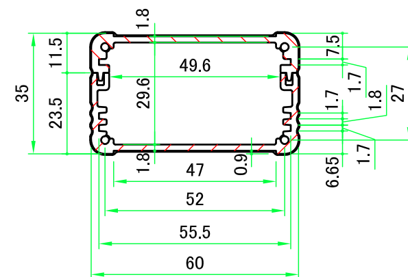
A-A ( 1 : 1.5 )
